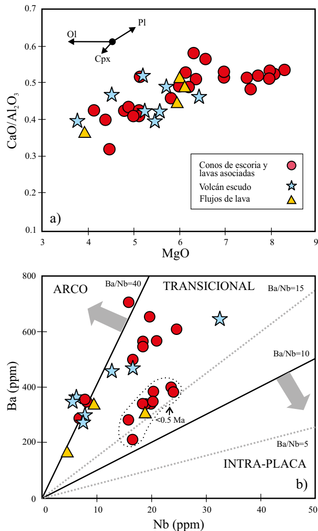
Figura 10 a) Relación de MgO vs. Ca/Al 2 O 3 para todas las muestras del CVAT. Se observan procesos de cristalización fraccionada de olivino para los basaltos, el traquibasalto y las traquiandesita basálticas, mientras que para las andesitas basálticas se observa cristalización fraccionada de clinopiroxeno. Modificado de Morra et al. (1997); b) concentraciones de Nb y Ba para las muestras del área de estudio. La mayoría de las rocas máficas caen en el campo transicional definido por D'Orazio et al. (2004).
