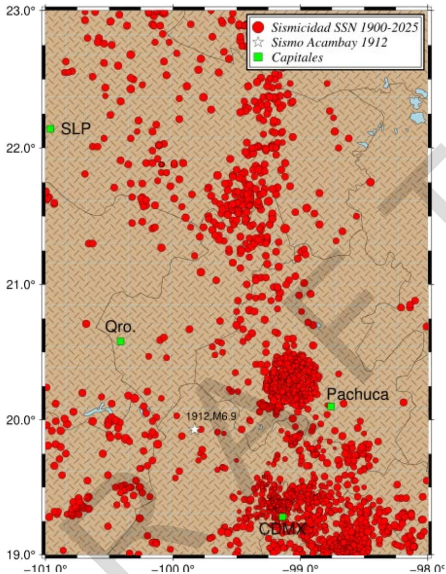
Figura 2. Sismicidad instrumental regional registrada por el SSN de enero de 1974 a febrero de 2025. La estrella indica el epicentro de los sismos de Acambay de 1912, los cuadros verdes las capitales de los estados. Las concentraciones de sismicidad hacia Hidalgo y Estado de México se deben a la existencia de al menos una estación sísmica en dicha zona (fuente: SSN, 2025).
