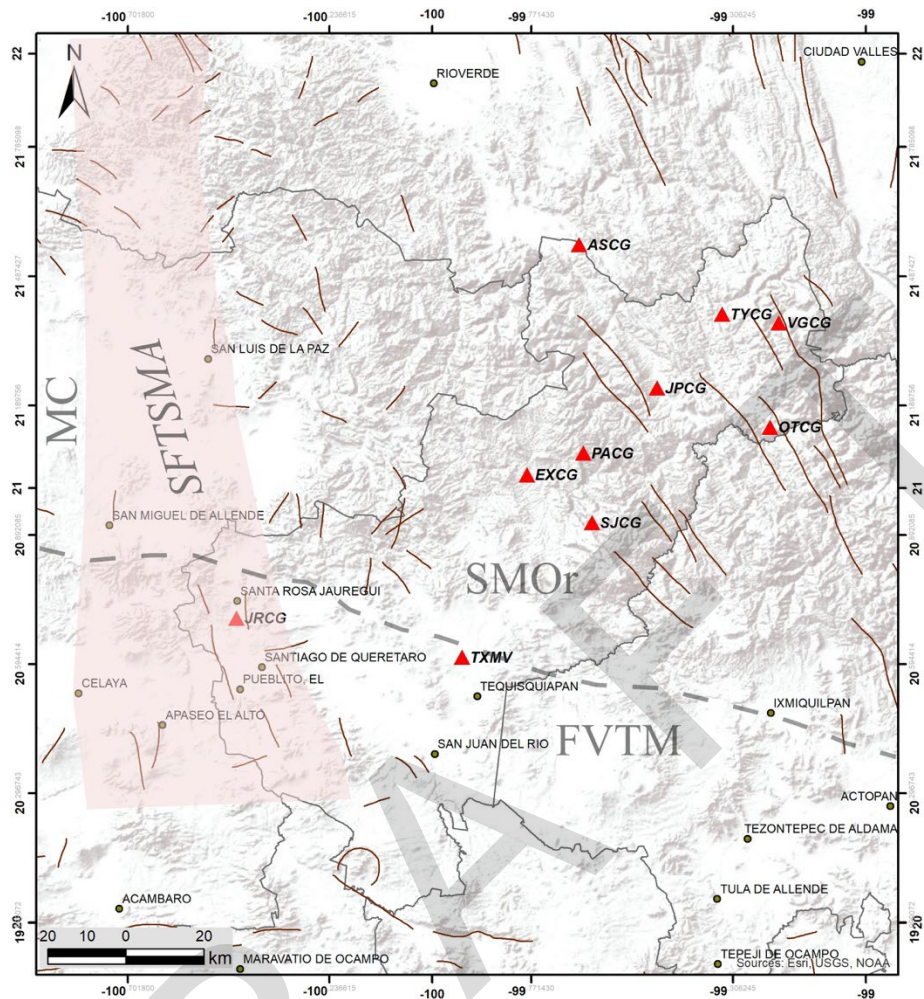
Figura 3. Provincias fisiográficas en el estado de Querétaro. SMOr: Sierra Madre Oriental (SMOr), FVTM: Faja Volcánica Transmexicana, MC: Mesa Central, SFTSMA: Sistema de Fallas Taxco San Miguel de Allende. Las líneas café indican las fallas en la región y los triángulos la ubicación de las estaciones de la Red Sísmica de Querétaro.
