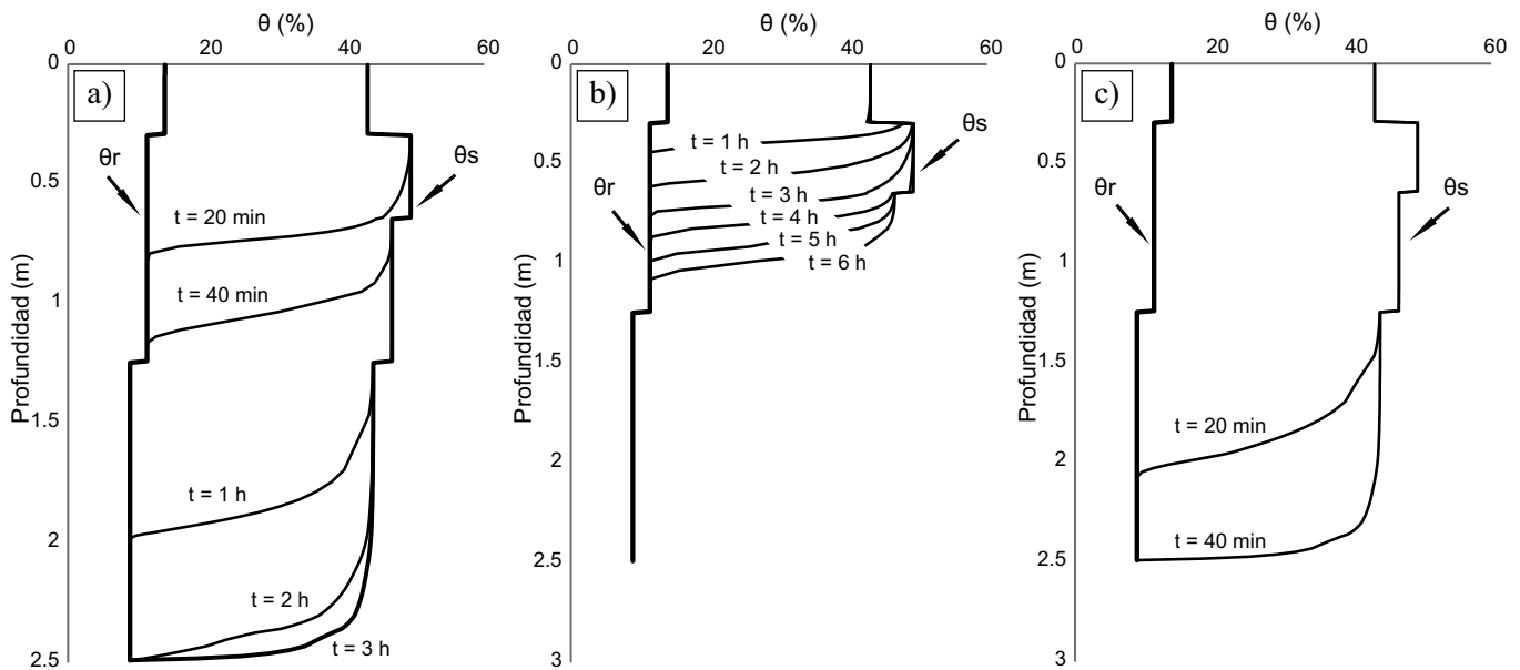
Figura 8. Resultados del análisis numérico. Sensibilidad de la conductividad hidráulica ( K_{sf} ): (a) K_{sf} medida en campo: 2.5–5 m \cdot d^{-1} , (b) K_{sf} un orden de magnitud menor (0.25–0.5 m \cdot d^{-1} ); (c) K_{sf} de un orden de magnitud mayor (25–50 m \cdot d^{-1} ).
