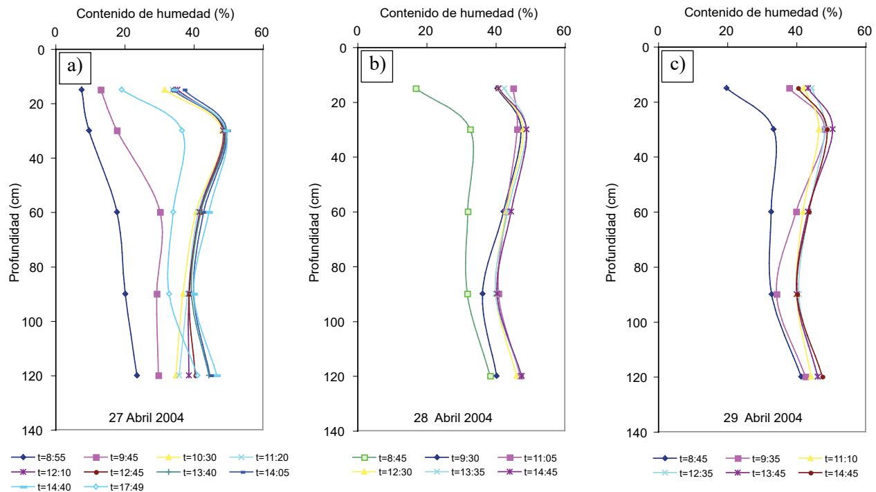
Figura 5. Respuesta en el contenido de humedad de los cinco sensores del electrodo de Refractometría en el Dominio del Tiempo (RDT) a las pruebas de infiltración, con la función de la Figura 4. Respuesta en los días a) 27 de abril, b) 28 de abril y c) 29 de abril de 2004.
